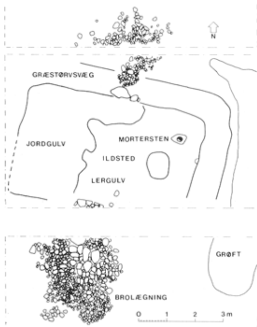
Fig. 5: Plantegning af hus 13 fra Heltborg byhøjen.
