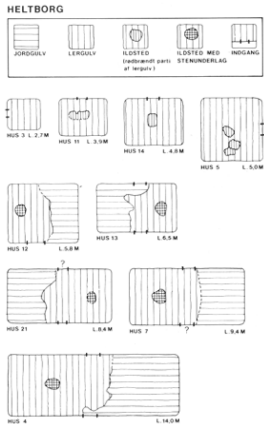
Fig. 2: Skematiserede grundplaner fra udvalgte huse.
