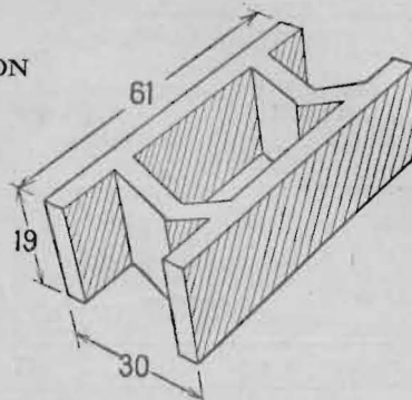
FUNDABLOK Betonstøbning uden Forskalling til 30 og 35 cm Murtykkelse
